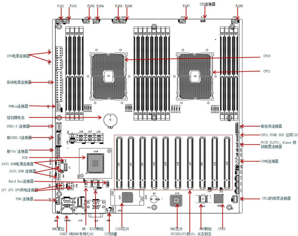
主板图 2-15
